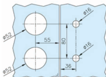
Glastür-Schlosskasten mit Drücker und Riegelaufnahme Öffnungsrichtung links, für Eurozylinder Lieferung exklusive Eurozylinder
