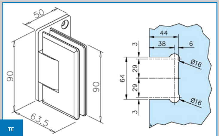
Türscharnier 14424
