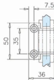
Glas/Wand Montage
