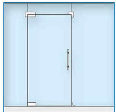
Montage-Set: Boden/Glas/Glas Art-Nr.: 792996068
