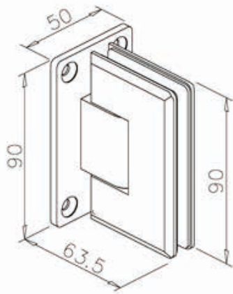
Türscharnier 12224
