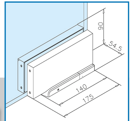
Hydraulischer-Beschlag
