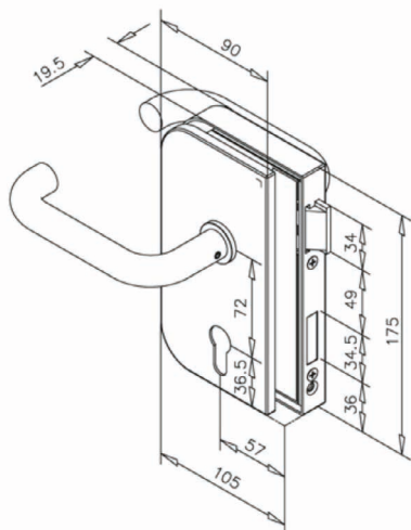
Glastür-Schlosskasten mit Drücker, Öffnungsrichtung rechts, für Eurozylinder Lieferung exklusive Eurozylinder
