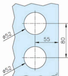
Glastür-Schlosskasten mit Drücker Öffnungsrichtung links, für Eurozylinder Lieferung exklusive Eurozylinder
